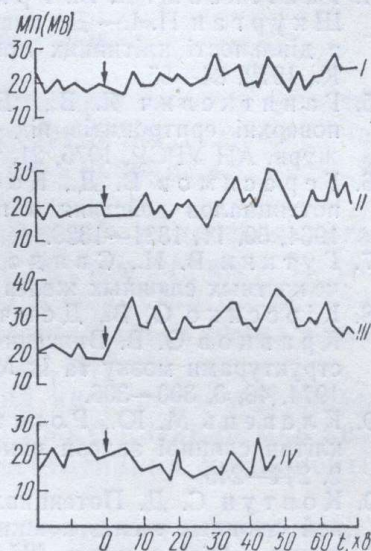
Динаміка змін МП клітин слинної залози молюска при перфузії розчинами ПАР.
